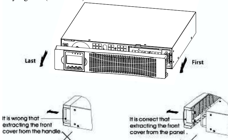
Gambar 5. Ambil penutup depan UPS
